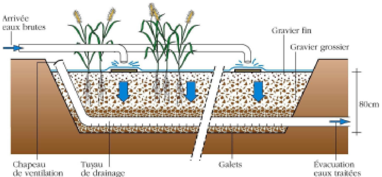
Figure 1 : coupe transversale d'un filtre à écoulement vertical
